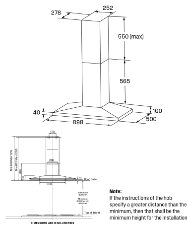
Canopy rangehood WRC914SD
